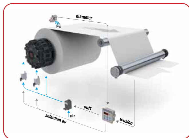
Applicazione su svolgitori con T-One SEL-XP Unwinder application with T-One SEL-XP
