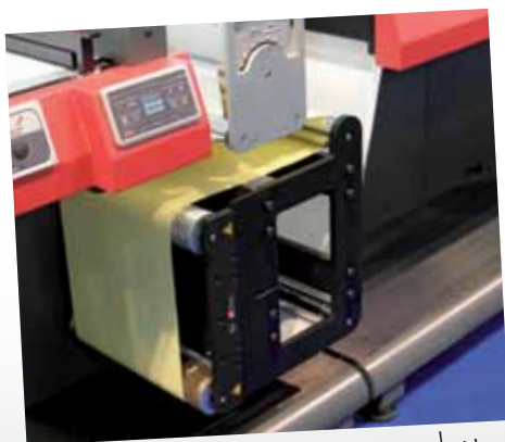
Guidanastro MWG.1D su macchina per etichette MWG.1D webguide on label machine
